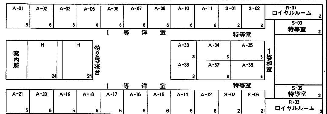
Aデッキ
